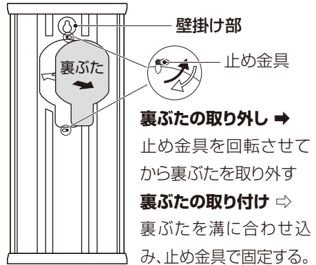
(裏面)
